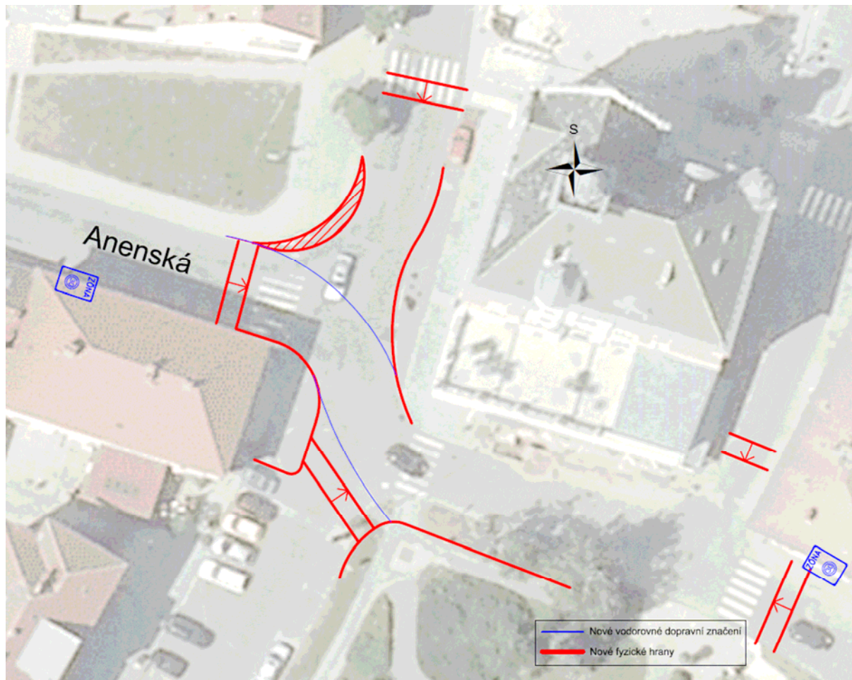
Obr. 27 – Návrh přestavby křižovatky ul. Národní třída x Anenská x Zámecká x Jánošíkova
