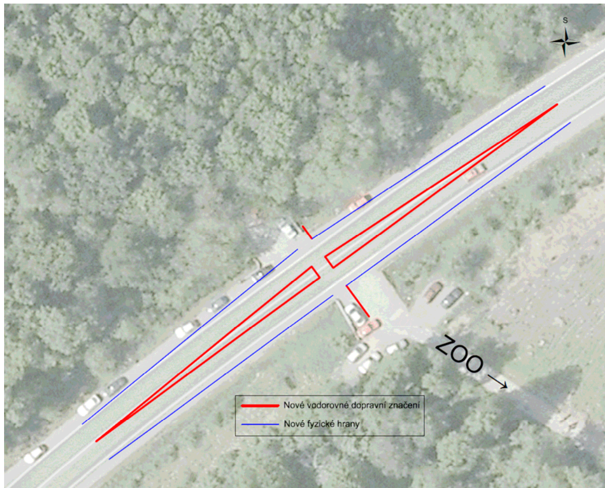
Obr. 38 - Vychýlení jízdních pruhů pomocí dělicího ostrůvku
