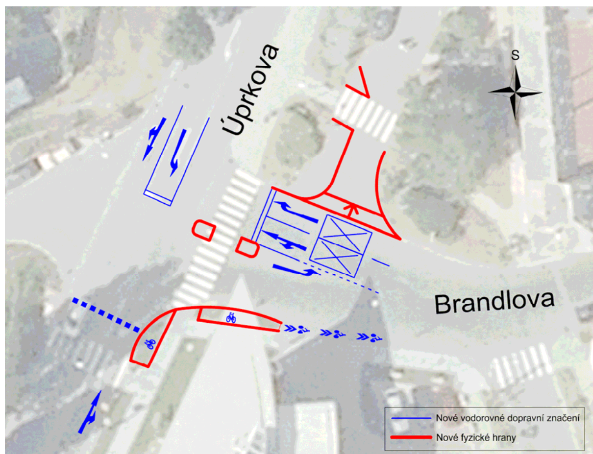
Obr. 30 – Návrh na řešení prostoru křižovatky Úprkova x Brandlova x Wilsonova
