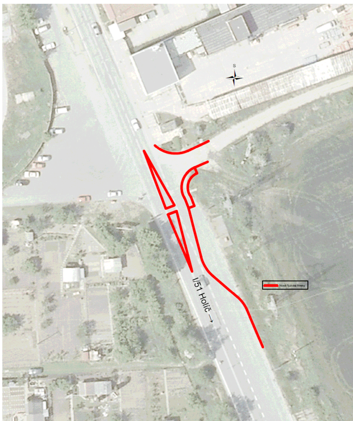
Obr. 26 – Návrh vjezdové brány na silnici I/51 ze směru od hranice se Slovenskem
